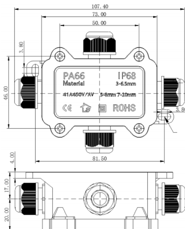
Dimensioni (mm)
