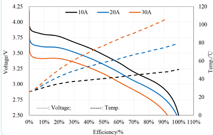
CURVE DI SCARICA
